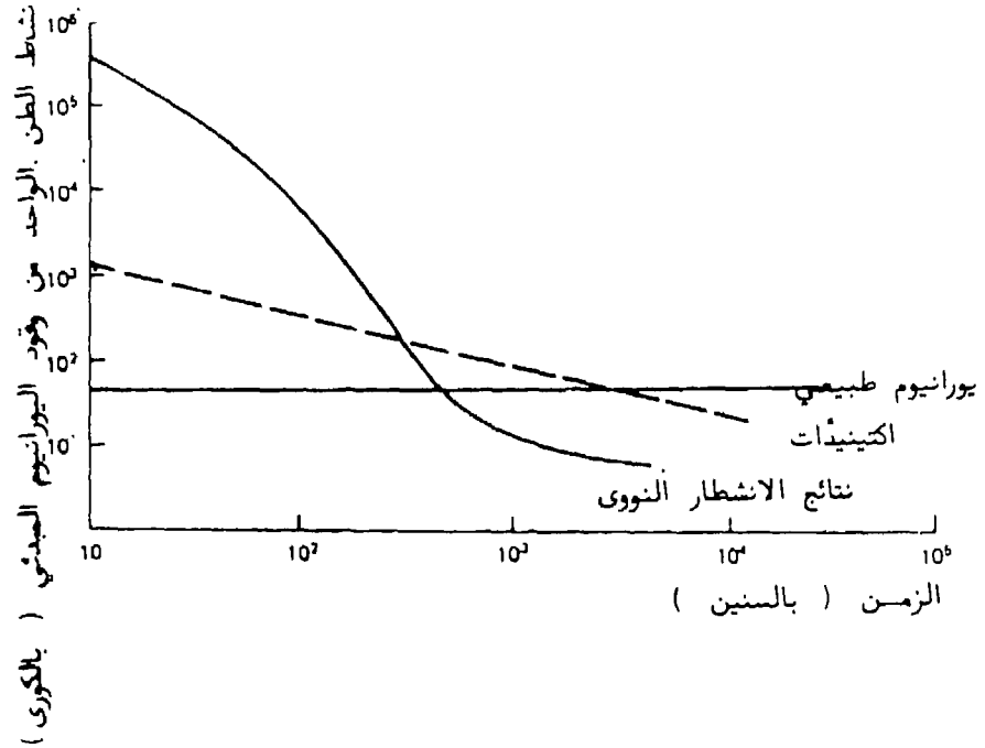
الشكل (9) رسم توضيحي لمناهج اضمحلال النشاط الإشعاعي لليورانيوم الطبيعي ، والاكينيدات ، ونواتج الانشطار النووي للمعروفة من المعاملات النووية .
